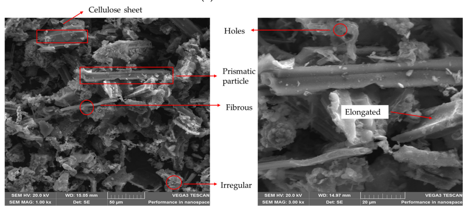
(b) SEM of SCBA
